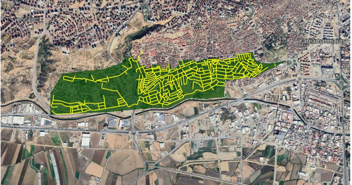
Şekil 4 Önerilen İçme Suyu Şebekesi
