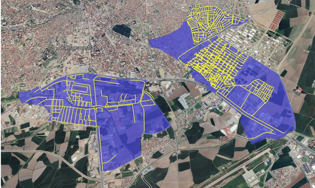
Şekil 4 Önerilen İçme Suyu Şebekesi
