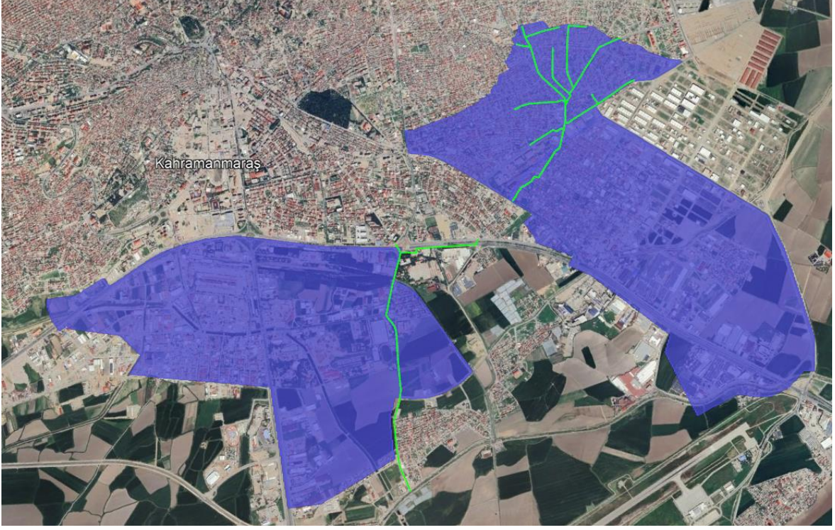
Şekil 5 Önerilen Yağmursuyu Ağı
