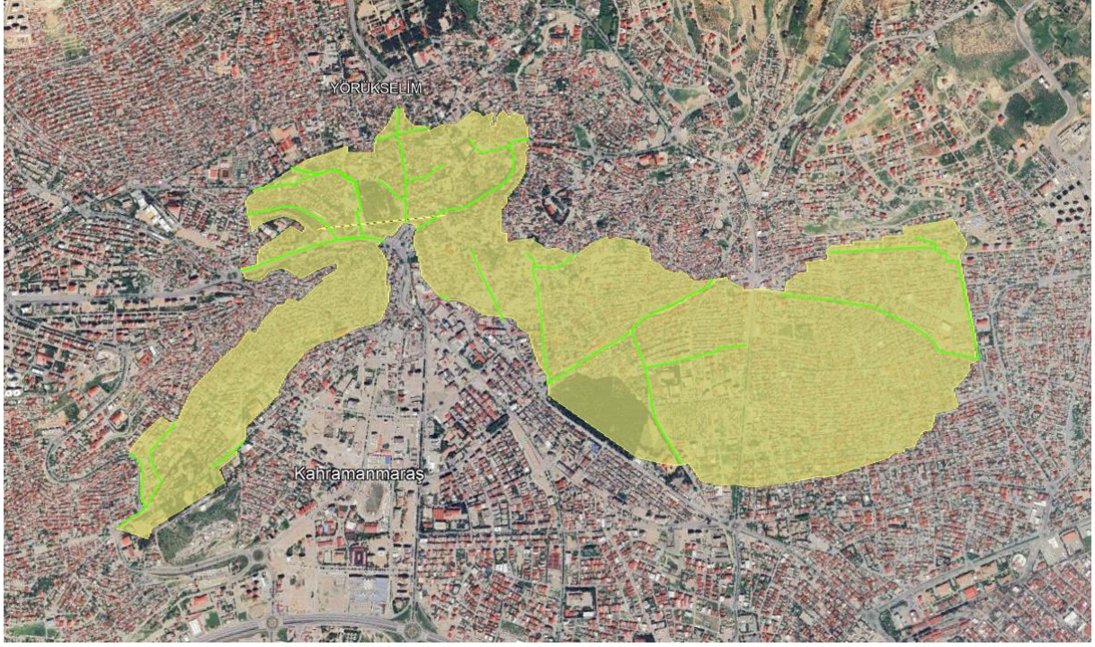
Şekil 5 Önerilen Yağmursuyu Ağı
