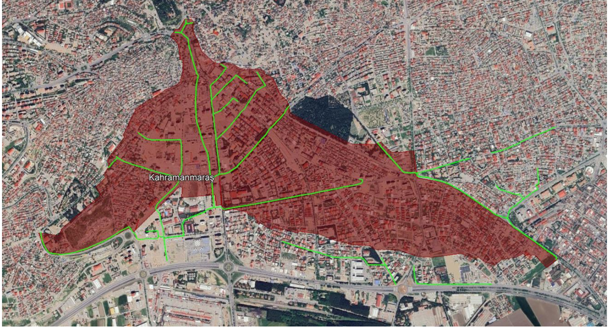
Şekil 5 Önerilen Yağmursuyu Ağı
