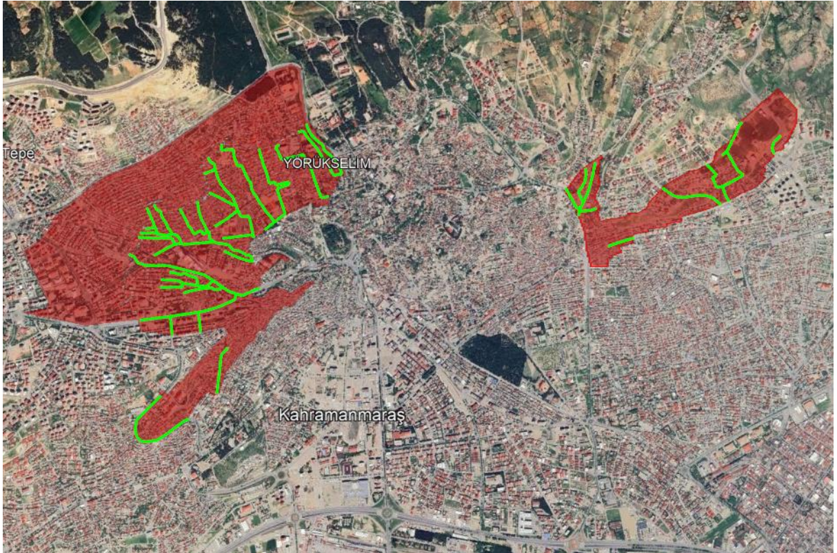
Şekil 5 Önerilen Yağmursuyu Ağı
