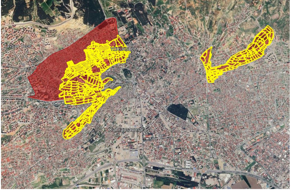
Şekil 4 Önerilen İçme Suyu Şebekesi
